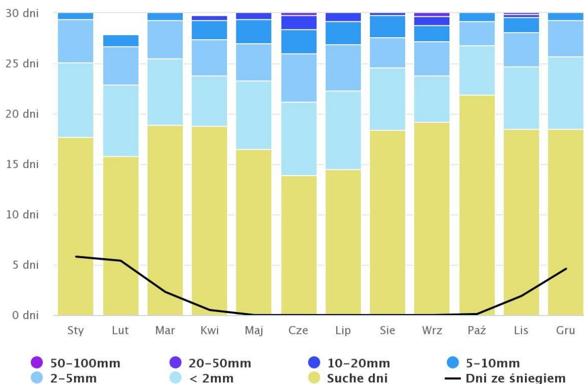
Ryc. 13. Średnie wartości opadów w roku dla analizowanego 30-lecia (na podstawie www.meteoblue.com ) w miejscowości Opatów
