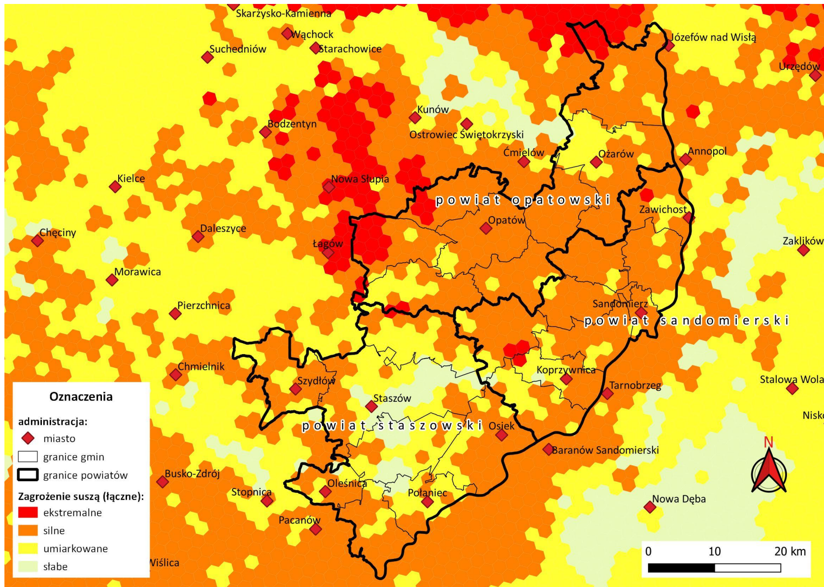
Ryc. 18. Łączne zagrożenie suszą na terenie analizowanych powiatów
