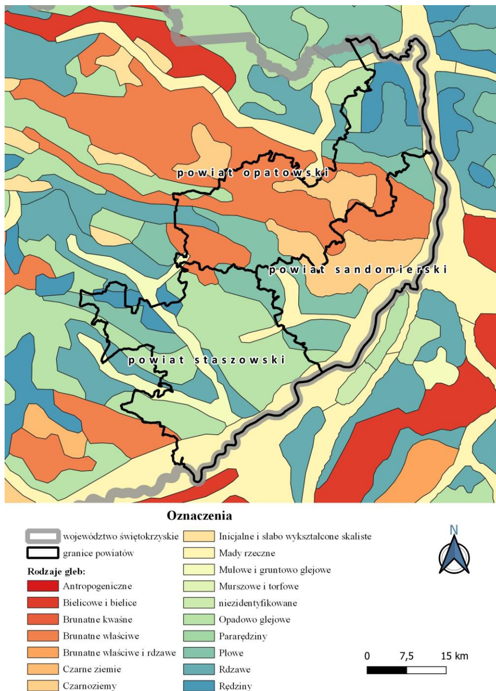
Ryc. 4. Zróżnicowanie gleb na obszarze analizowanych powiatów
