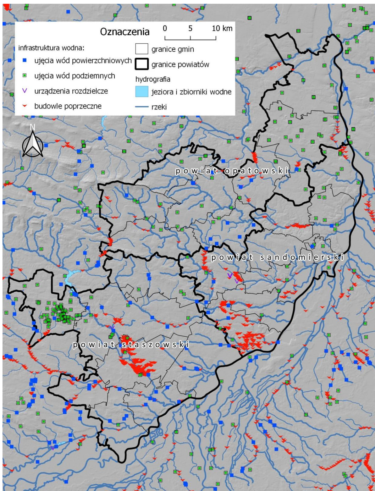
Ryc. 19. Wybrane elementy infrastruktury wodnej na terenie analizowanych powiatów
