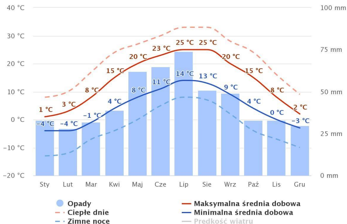
Ryc. 12. Rozkład średnich temperatur i opadów analizowanego 30-lecia (na podstawie www.meteoblue.com ) w miejscowości Opatów
