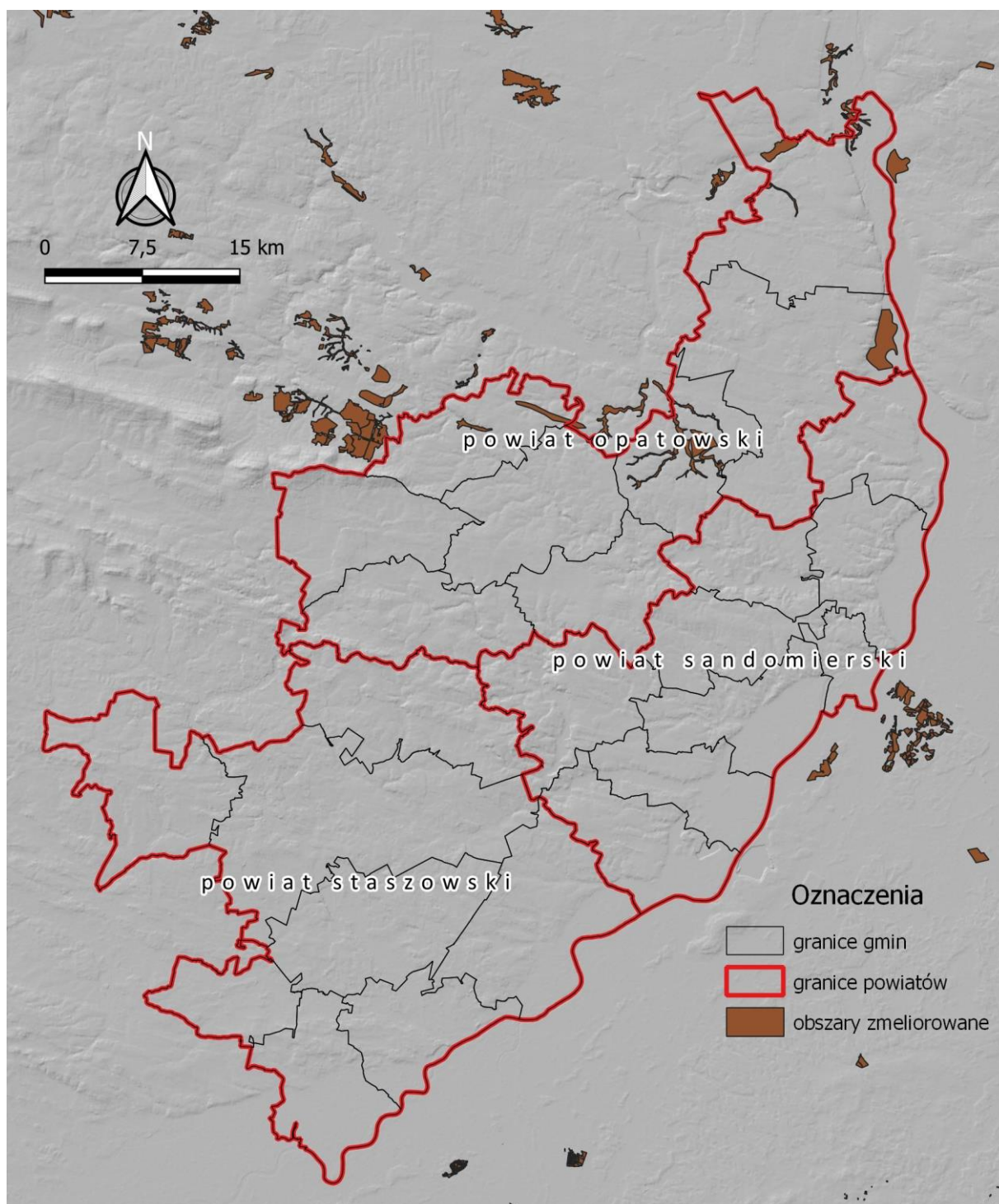
Ryc. 8. Obszary zmeliorowane w granicach analizowanych powiatów
