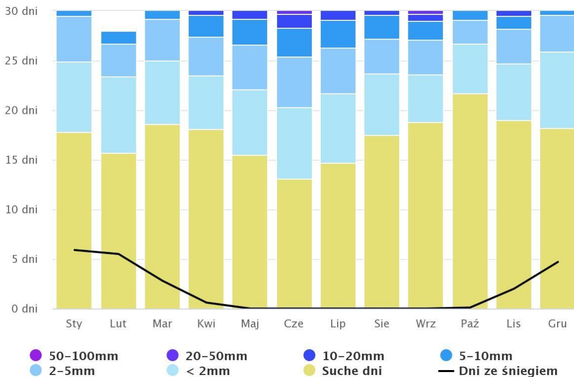
Ryc. 15. Średnie wartości opadów w roku dla analizowanego 30-lecia (na podstawie www.meteoblue.com ) w miejscowości Staszów
