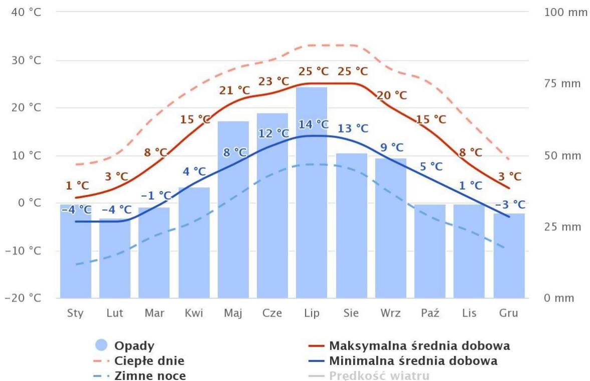
Ryc. 10. Rozkład średnich temperatur i opadów analizowanego 30-lecia (na podstawie www.meteoblue.com) w miejscowości Sandomierz
