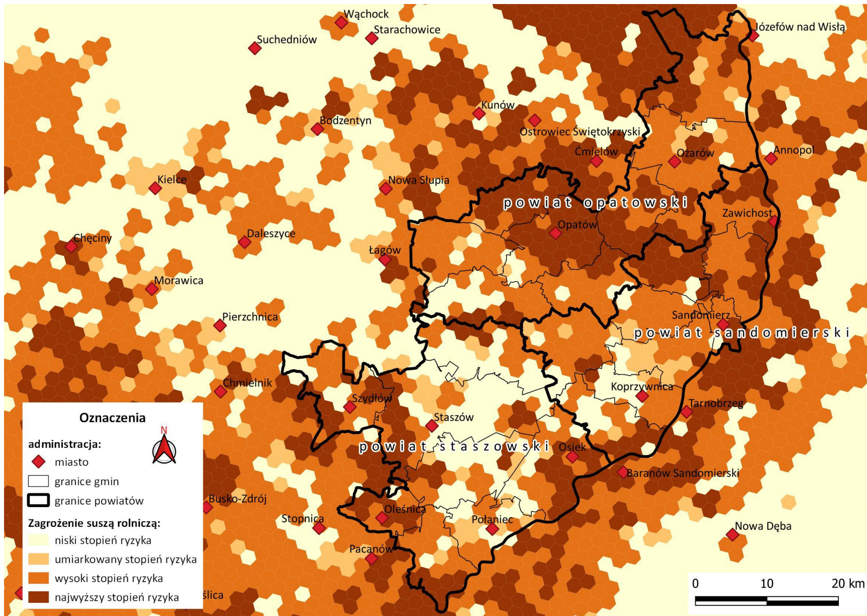
Ryc. 17. Zagrożenie suszą rolniczą na terenie analizowanych powiatów
