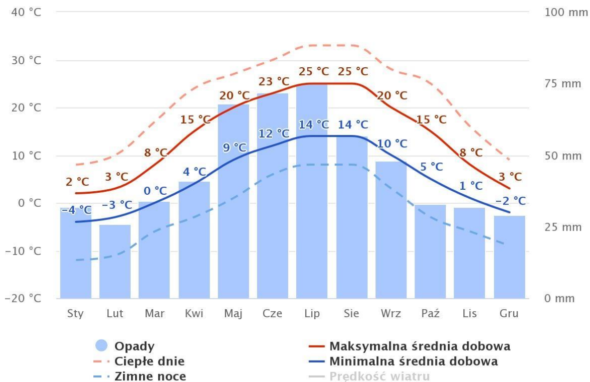
Ryc. 14. Rozkład średnich temperatur i opadów analizowanego 30-lecia (na podstawie www.meteoblue.com ) w miejscowości Staszów
