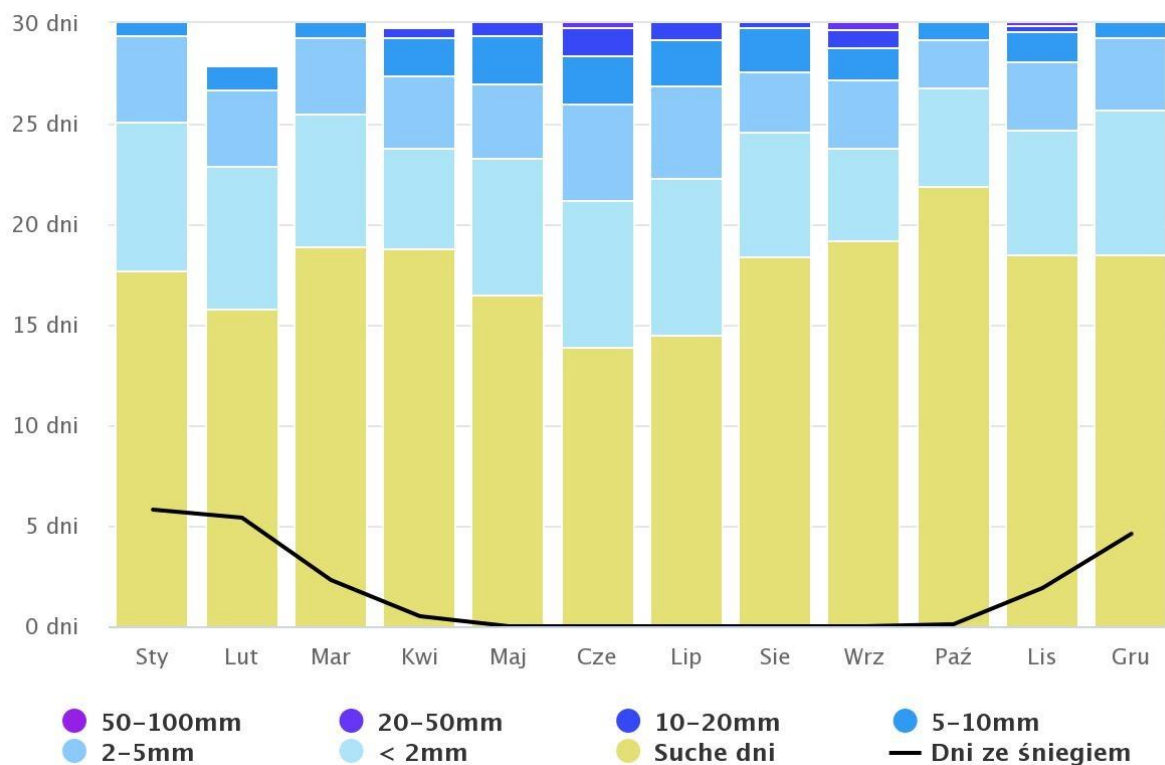
Ryc. 11. Średnie wartości opadów w roku dla analizowanego 30-lecia (na podstawie www.meteoblue.com) w miejscowości Sandomierz
